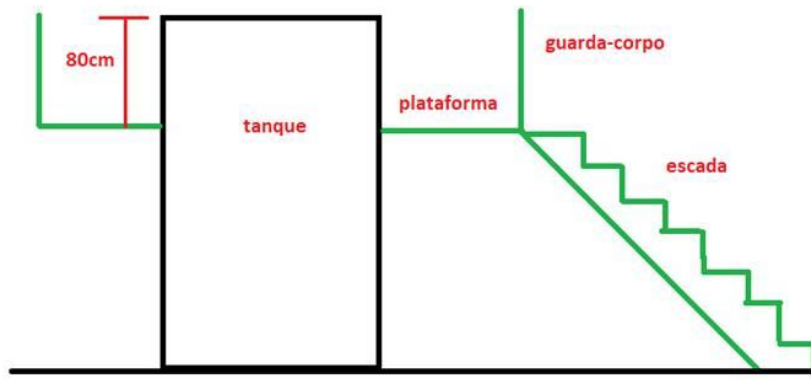
Figura 2 - Alturas do piso da plataforma e layout de referência da escada
